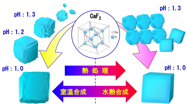
溶液反応プロセスによる \text{CaF}_2 ナノクリスタルの生成機構
