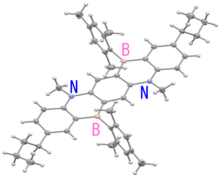
窒素とホウ素を使った 緑色に光る化合物
