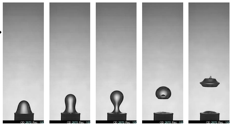
撥水面から離脱する気泡の様子
