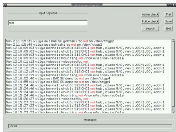
検索可能暗号化ログの検索の様子
