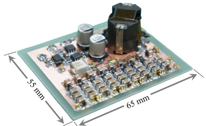
研究室で開発した蓄電池用 パワーエレクトロニクス回路
