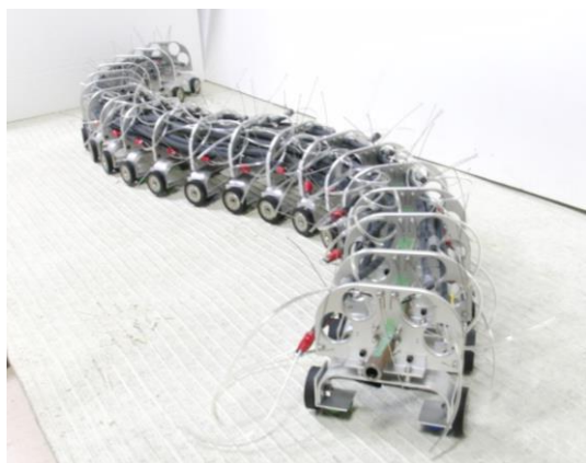
人工筋肉を持つヘビロボット
