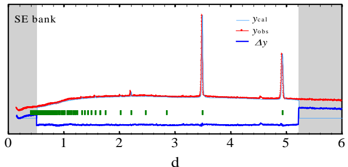
中性子回折データの例
